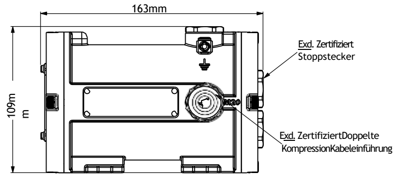
SEITENANSICHT
