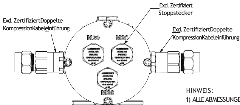
RÜCKANSICHT
