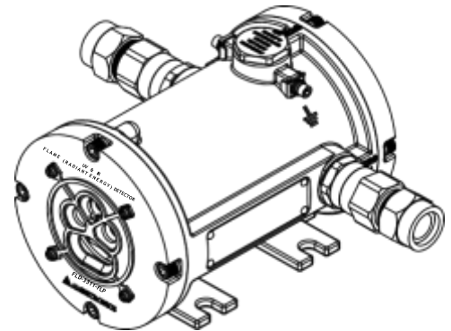
ISOMETRISCHE ANSICHT
